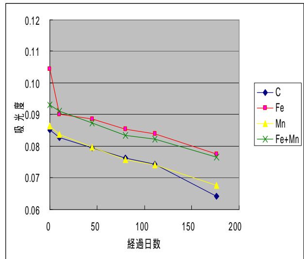
Fig.3 樽貯蔵後の麦焼酎のビン内での着色度の変化 (480nm)
