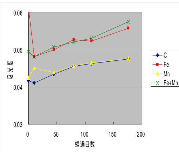
Fig.2 樽貯蔵後の麦焼酎のUVカットしたビン内での着色度の変化 (480nm)
