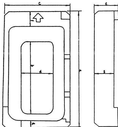
図3 上型発泡模型の寸法測定位置
