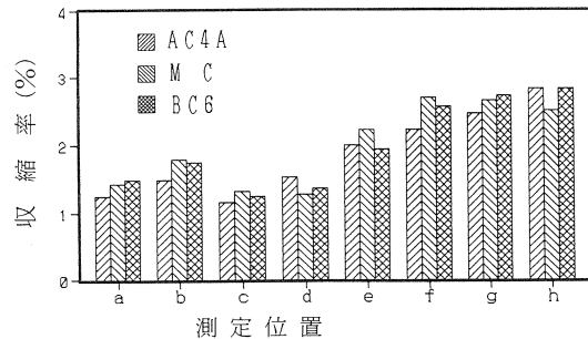
図6 模型に対する各測定点の収縮
