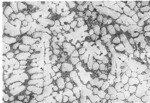
写真2 MCの鑄造組織
