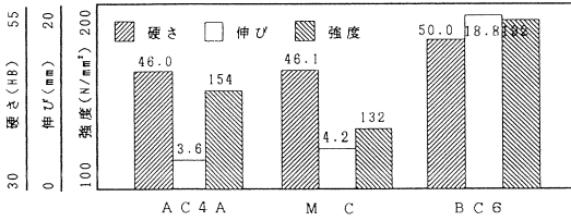
図8 各材質の機械的性質
